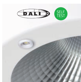
/EMDI DALI / Self test EM Integral ILEM
